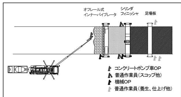
図-2 機械編成
