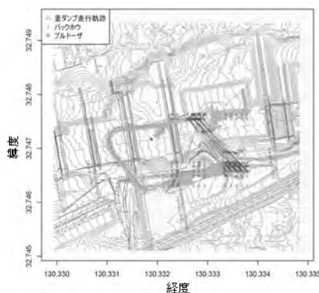
図-15 各建設機械の走行軌跡、土量
