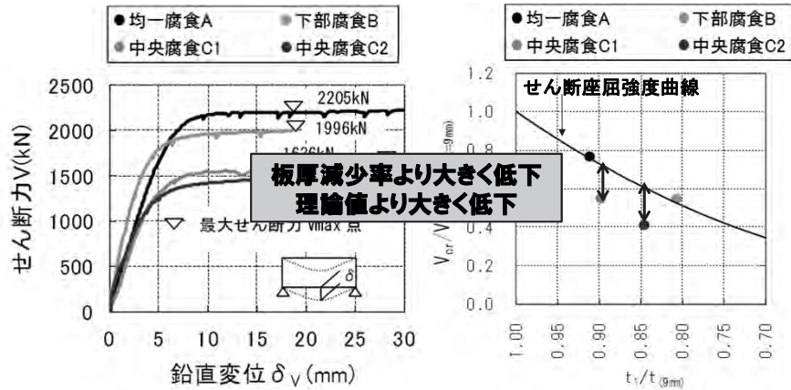
均一腐食A t_0=8.13\text{mm}
