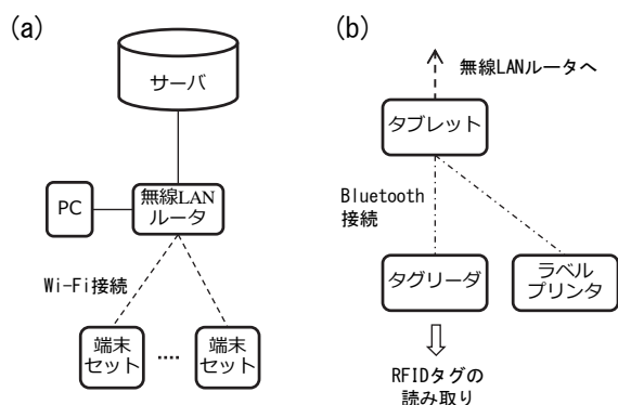
図-6 (a) 特定拠点で運用する際の最小システム構成図。(b) (a) の端末セットの詳細図。
