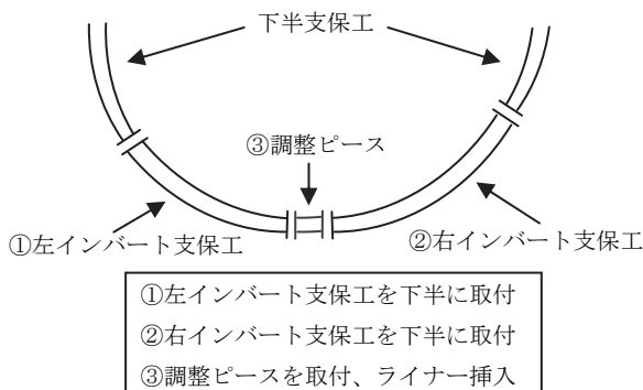
図-9 従来方式での建込手順
