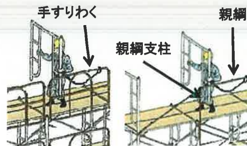
安全帯取付け設備の例
