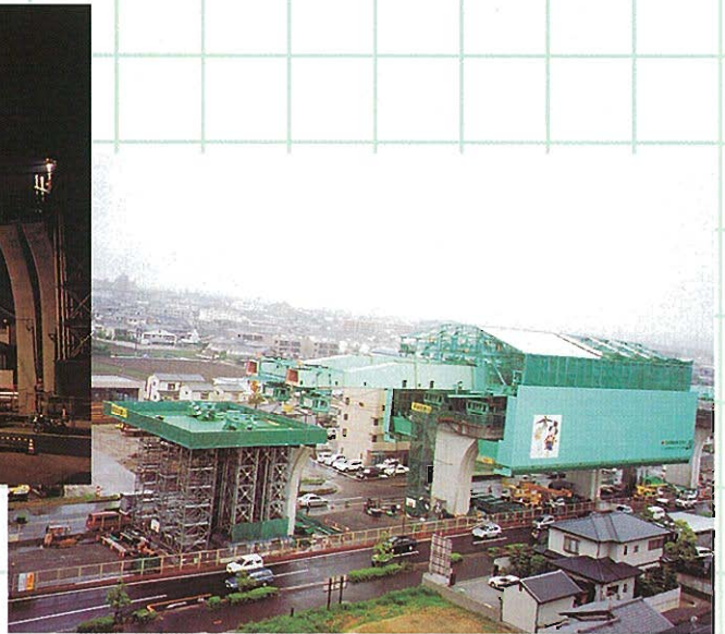
⇩後退前の大型移動支保工(左は仮受けベント)
