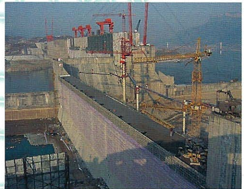
⇨仮締切ダムの上流側面⇨
