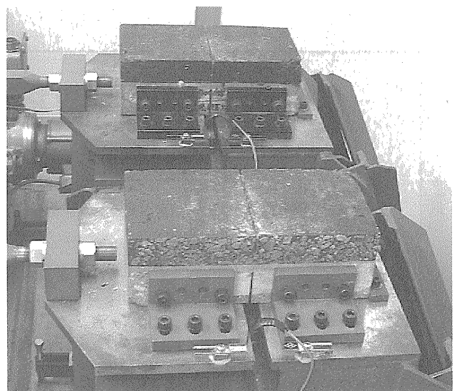
写真-3 ひび割れ負荷試験状況
