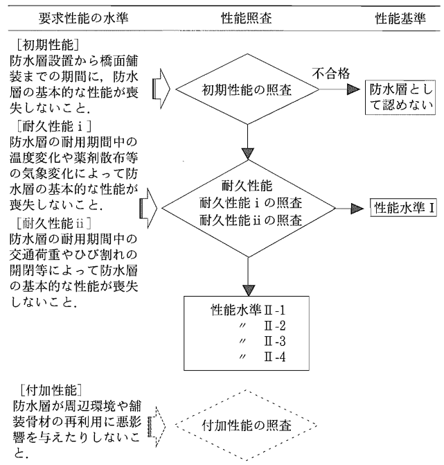
図-1 防水工の性能評価のフロー
