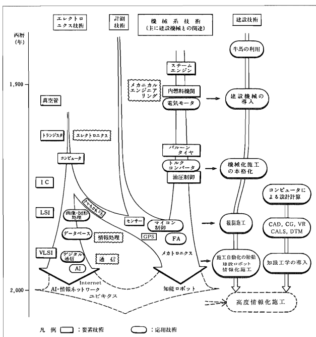
図-1 建設機械の進化
