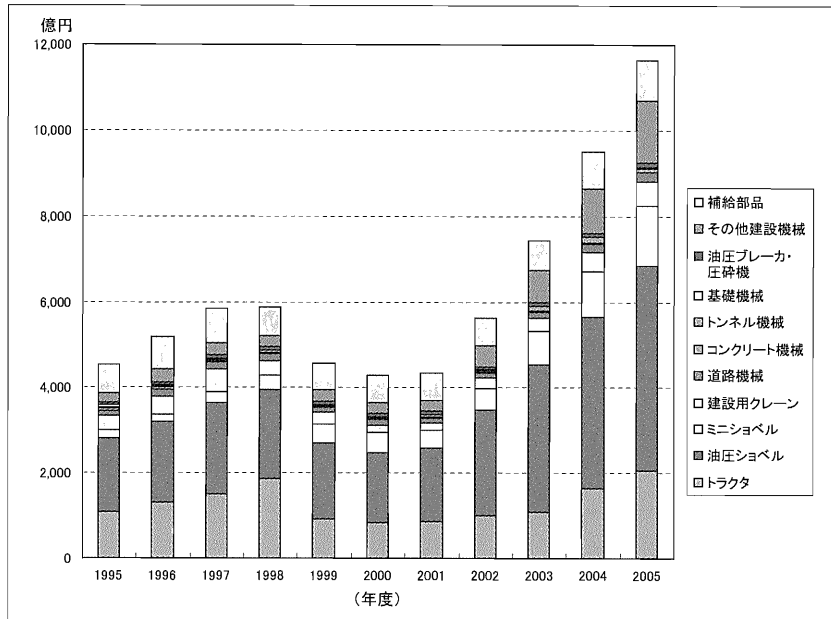
図-4 建設機械別海外出荷金額
