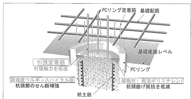
図—1 CTP工法概念図
