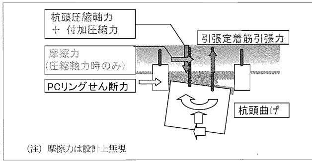
図-2 CTP 工法における力の伝達メカニズム
