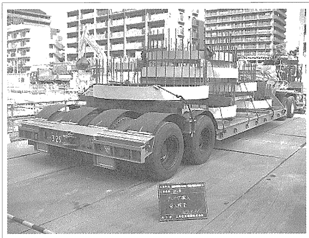
写真—4 PCリングの搬入
