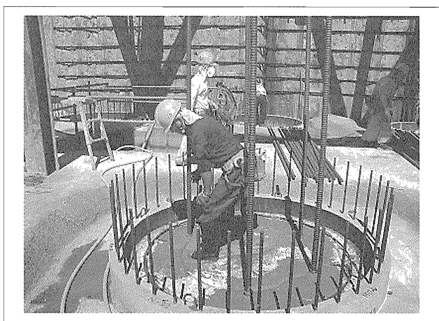
写真-10 引張り定着筋の挿入
