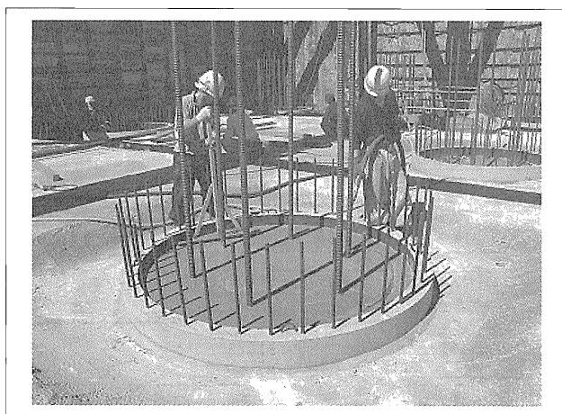
写真-11 杭頭接合部へのモルタル流込み
