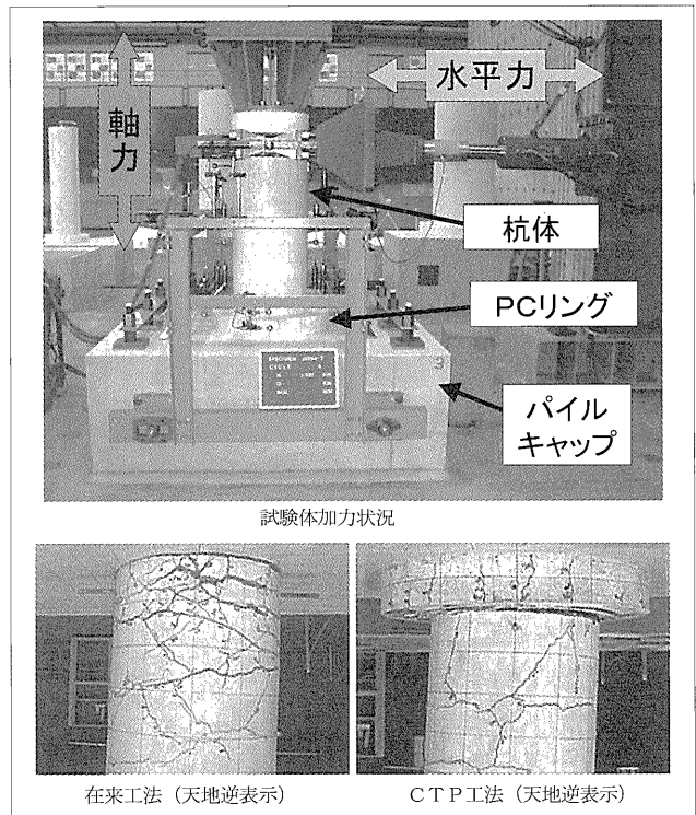
写真-1 杭頭接合部の曲げせん断実験
