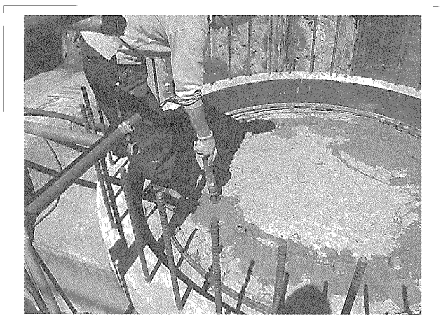
写真-9 シース内へのモルタル充填
