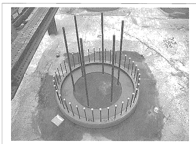
写真-12 杭頭部への発泡ポリエチレン設置
