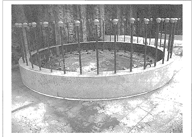
写真—6 PCリング下面の目詰め
