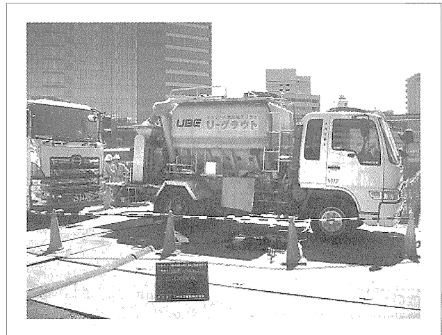
写真—7 ローリ車によるモルタル製造
