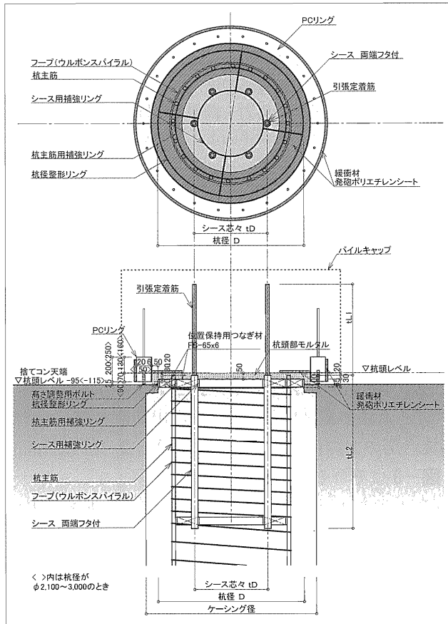
図-3 CTP 工法 杭頭断面図
