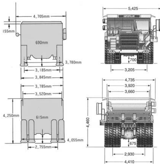
図一 車幅寸法図比較 (773Bと773F)
