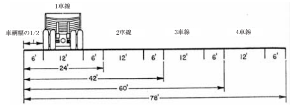
図二 米国鉱山局の車線幅員基準
