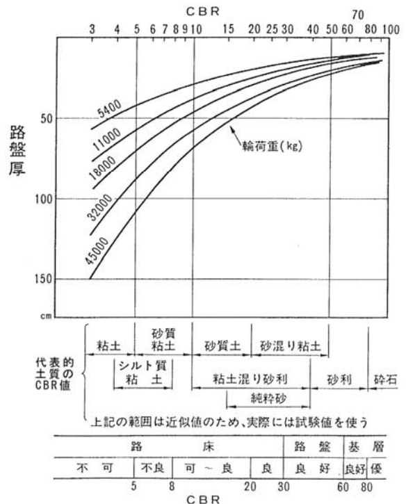
図—9 土の分類と CBR カーブ
