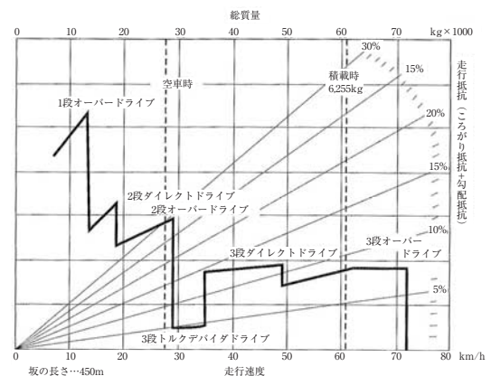
図-7 ブレーキ性能曲線
