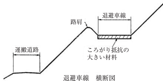
図—11 退避車線
