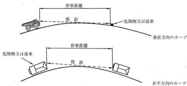
図-5 停車距離と視距
