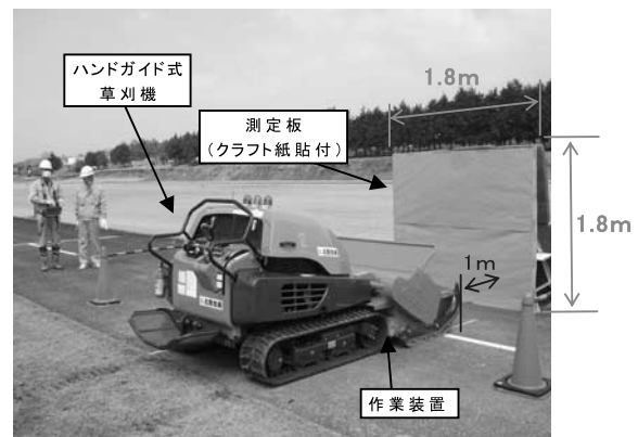
写真—2 実験装置の配置状況
