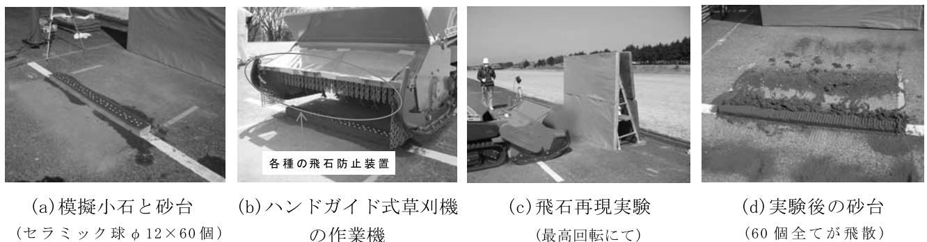
写真—3 飛石の再現実験
