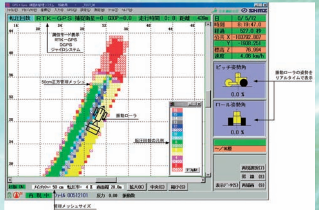
⇨ 4：GPS 締固め管理システムの振動ローラ搭載モニタリング画面
