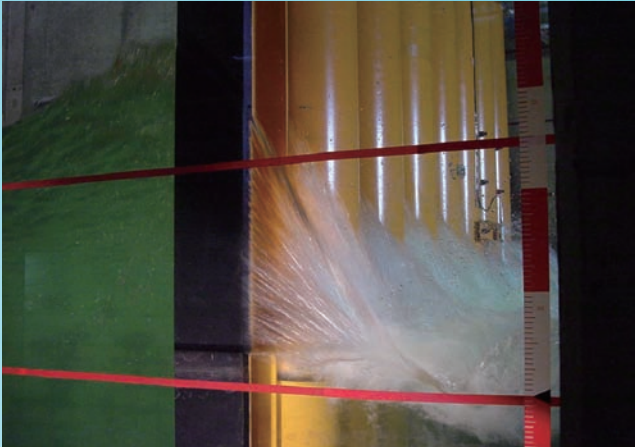
⇨水理模型実験（津波対象波・側面より）
