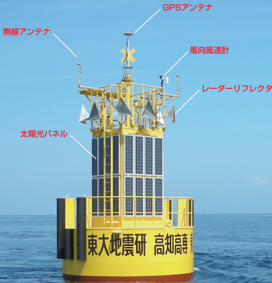
高知県室戸岬西方沖GPS津波計
