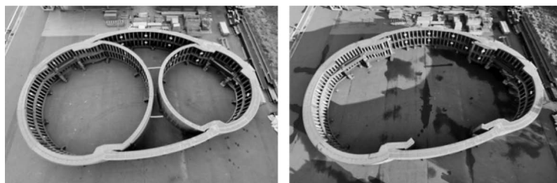
写真—1 アーチセグメント仮組
