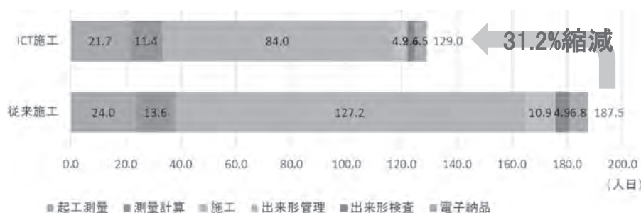
図—2 ICT土工の効果
