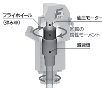
写真二 フライホイール式オーガ
