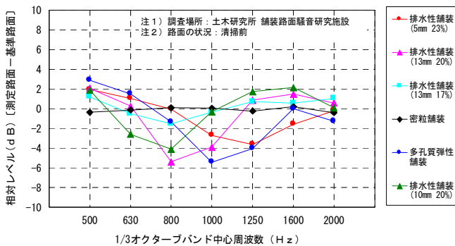
図-4 舗装構造別の吸音効果
