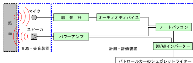
図－3 システムの機器構成図
