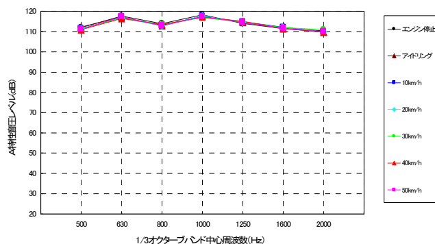
図－2 音源・受音装置の反射音測定
