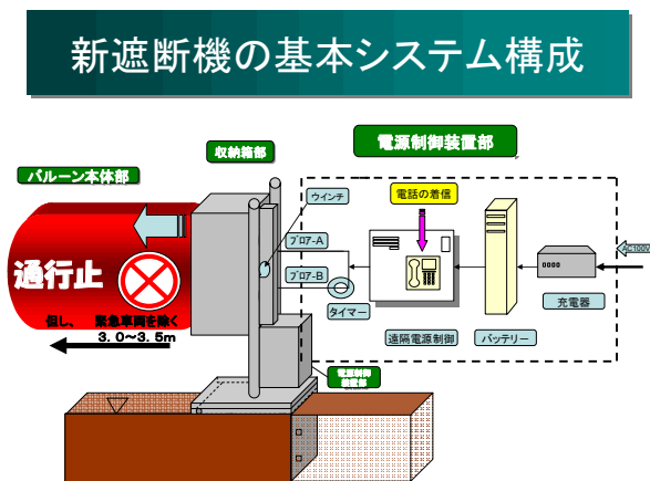
図ー２ 新遮断機の基本システム構成イメージ
