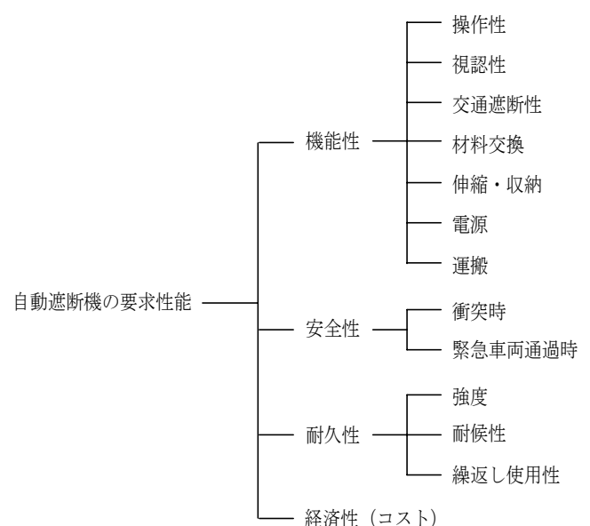
図ー３ 新遮断機に要求される性能
