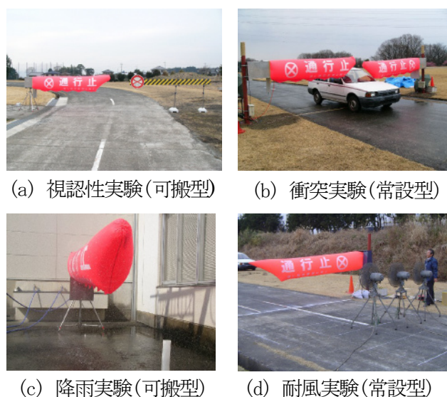
写真ー2 構内での試作機を用いた 性能確認実験状況
