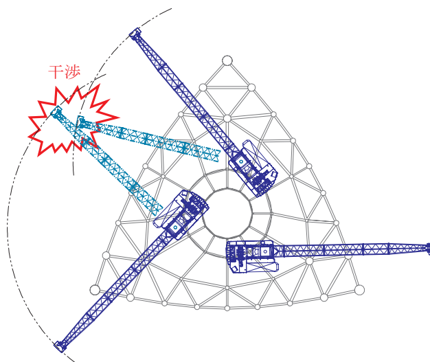
図-3 暴風時の問題点と塔体平面図
