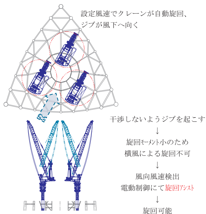
図-4 暴風時の改善点：「旋回アシスト」
