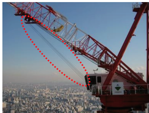
写真-1 あおり防止装置
