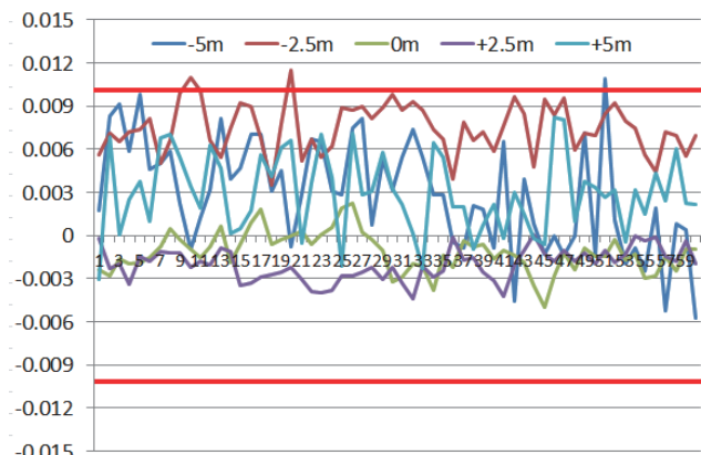
図-9 発光器から 250m 地点の観測結果
