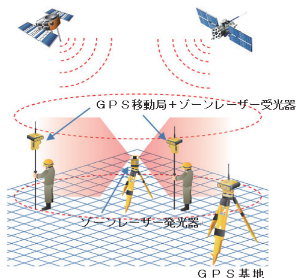
図-1 高さ補正装置(mmGPS)システム
