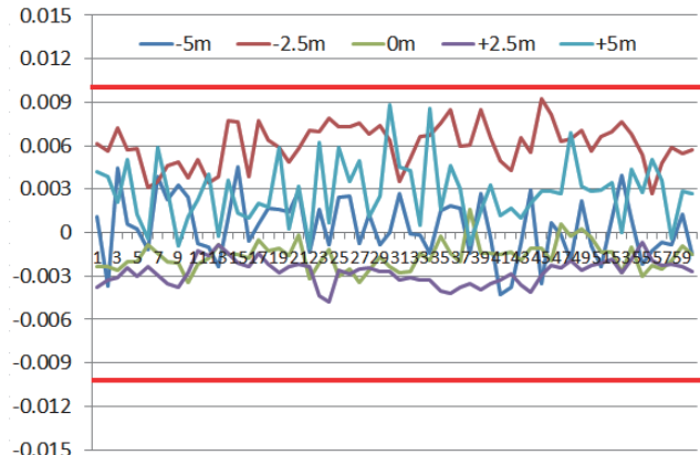
図-8 発光器から 200m 地点の観測結果
