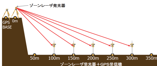
図-3 高低差-2.5m、-5m 観測方法
