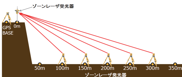
図-4 高低差+2.5m、+5m 観測方法
