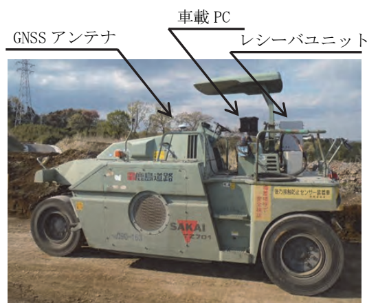
写真-3 VRS-RTK 機器構成
