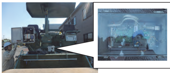
写真-8 慣性センサ機器構成
