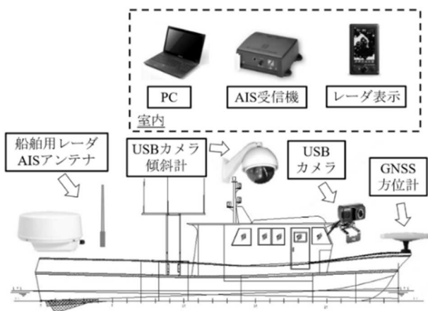
図-7 交通船への機材設置状況
