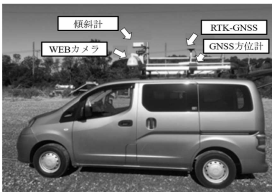
図-3 機材設置状況
