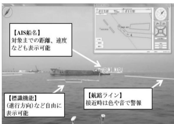
図-8 システム画面(海上試験時)
