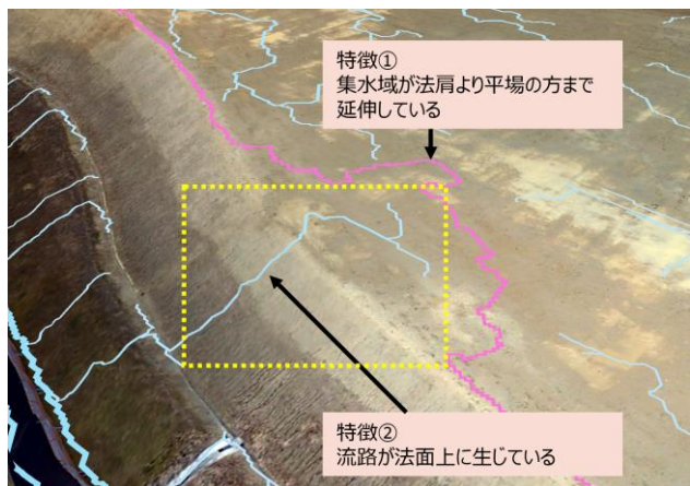
図-3 法面損傷リスクの特徴
