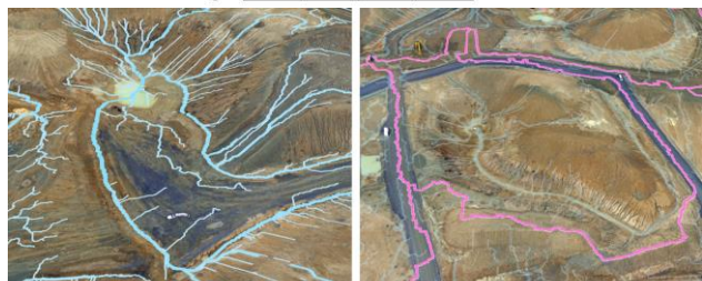
図-2 雨水表層流解析の結果（2024年2月19日地形）
