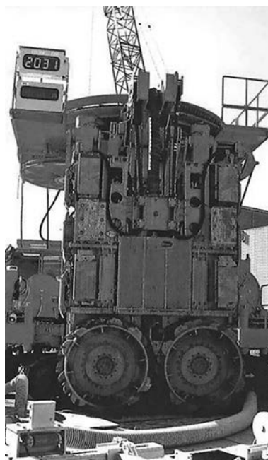
写真—4 BMX 掘削機
