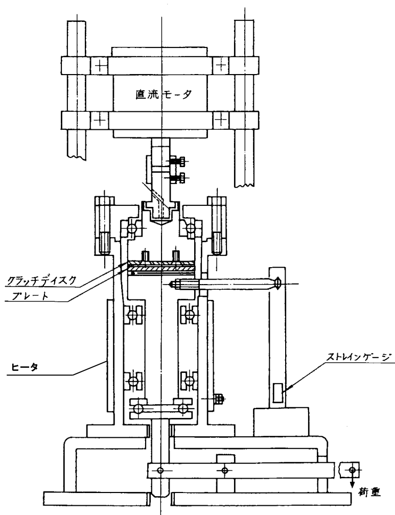
図5 マイクロクラッチ試験装置
