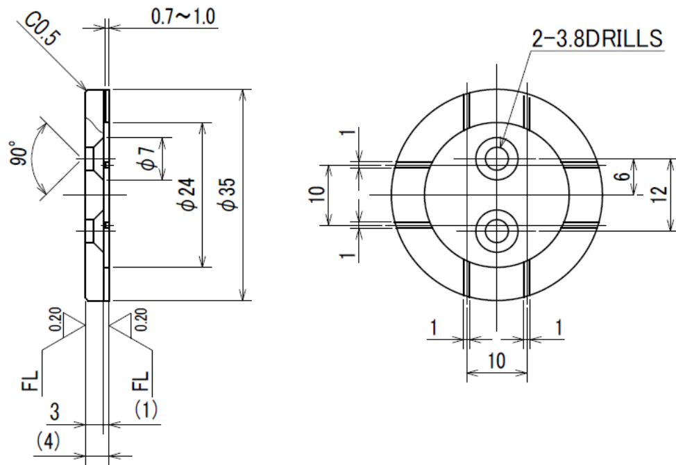
図 6 (a) クラッチディスク (SD1795-S)
