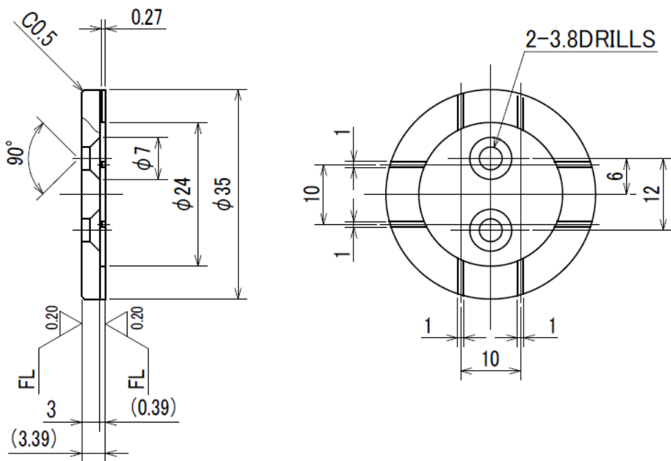
図 6 (b) クラッチディスク (NW-461E)
