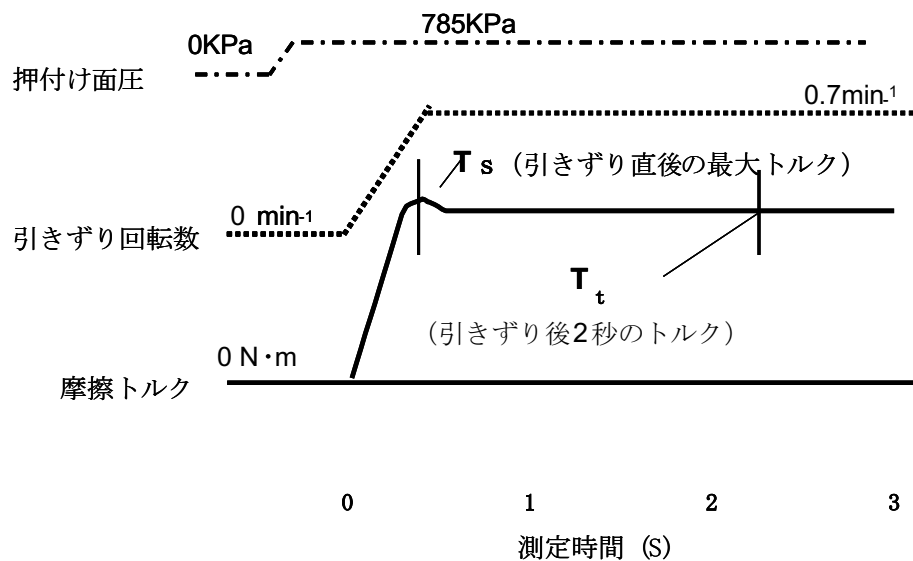
図4 静摩擦試験 (測定例)
