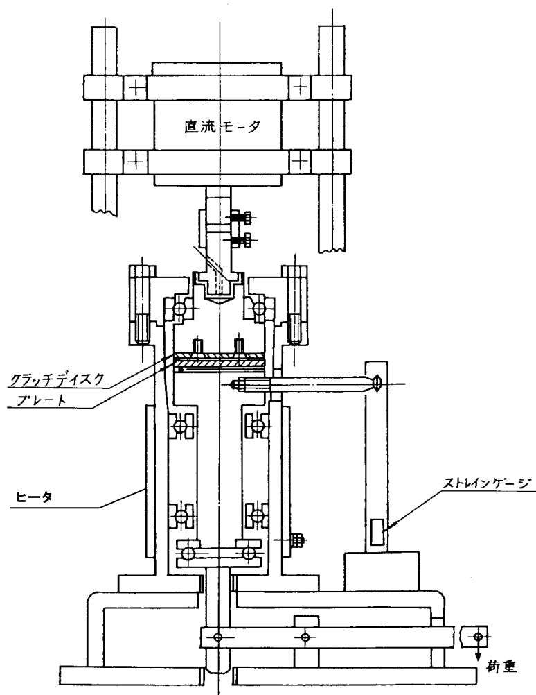
図 5 マイクロクラッチ試験装置
