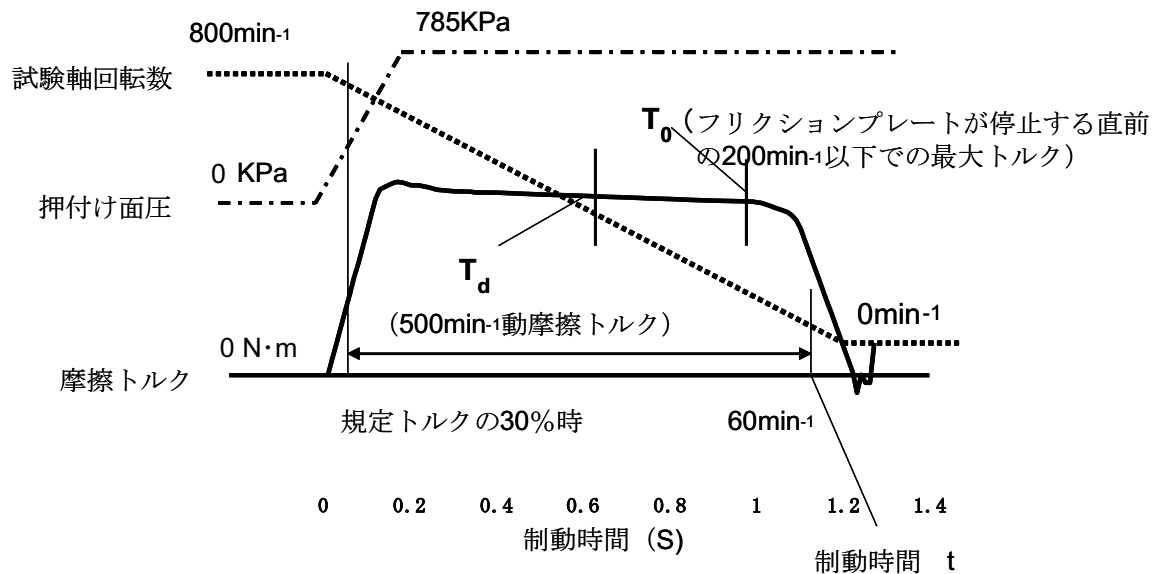
図3 動摩擦試験 (測定例)
