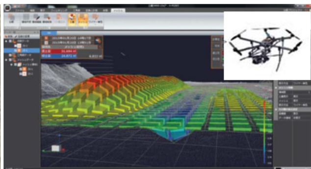
UAV 計測とソフトウェアによる点群処理と数量算出
