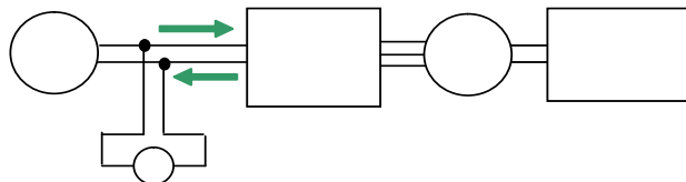
図 4 電力量計を用いた外部電力消費量測定方法の例
