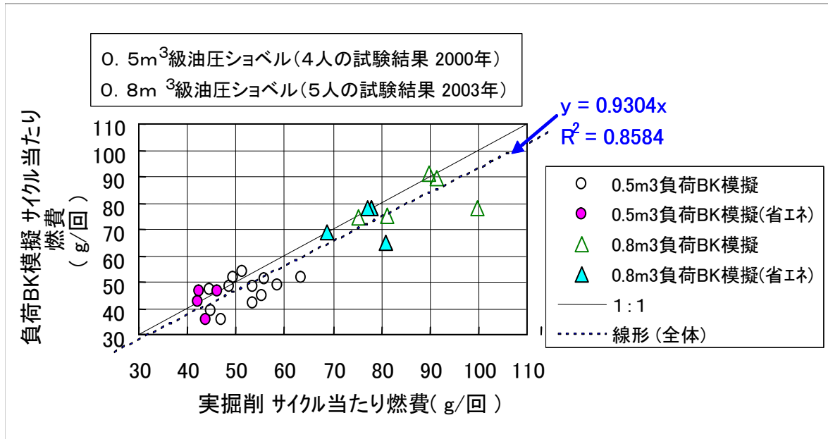
解説図 2 実掘削と模擬動作（負荷バケット付き，油圧負荷なし）との相関
