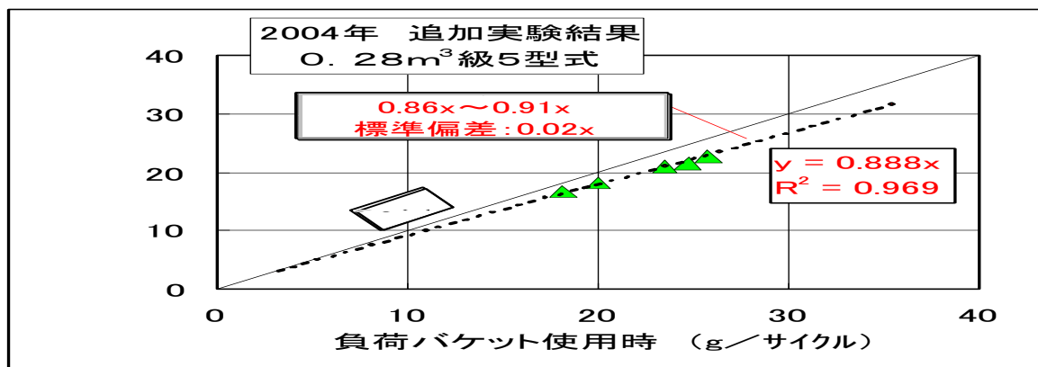
解説図 3 負荷バケットと空バケットとの相関
