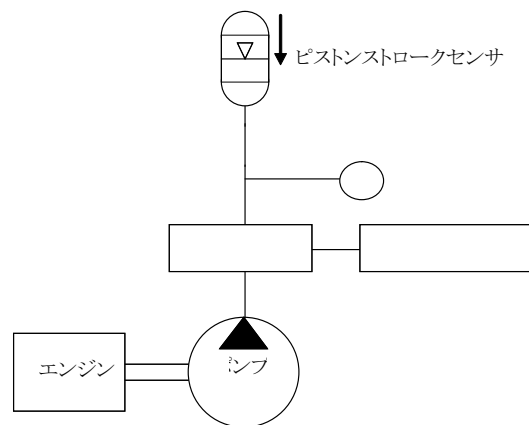
b) 圧力系と動力用アキュムレータの内部容量検出用ピストンストロークセンサとを用いた測定方法の例
