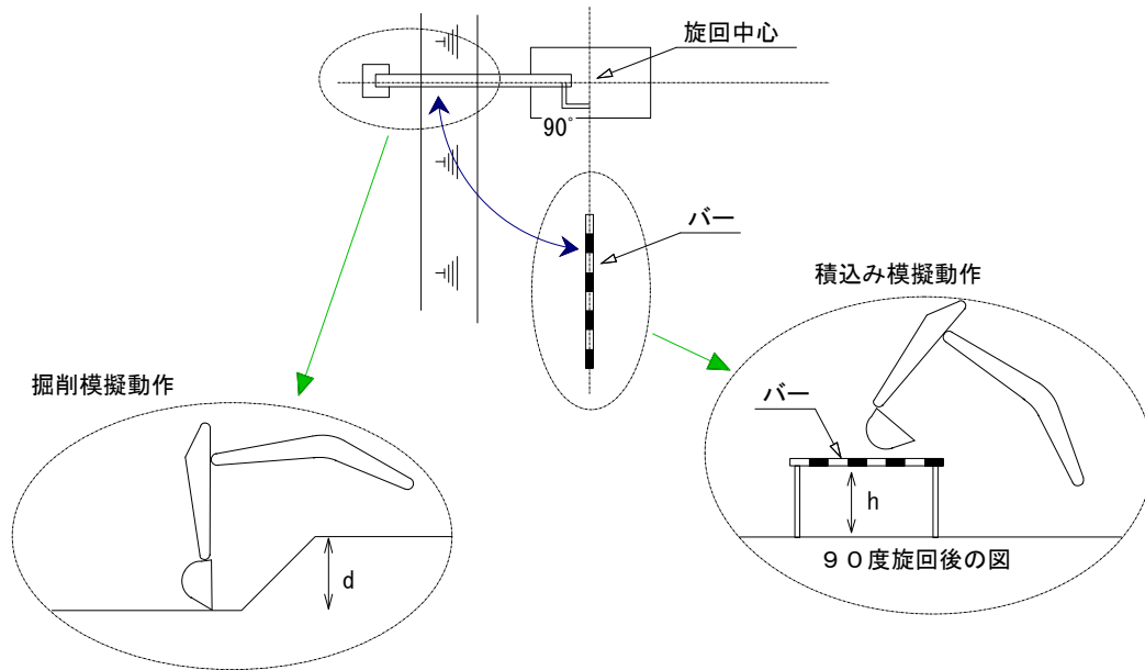
図 11 掘削・積み込み動作試験場
