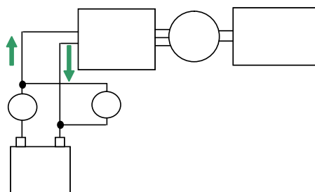
図 6 電流計と電圧計を用いた蓄電装置のエネルギー変化量測定方法の例
