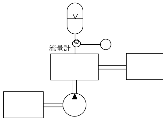
a) 圧力計と流量計とを用いた測定方法の例
