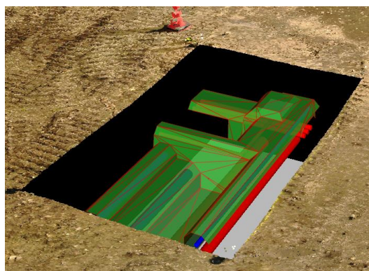
図-6 埋設管保護データの配置状況
