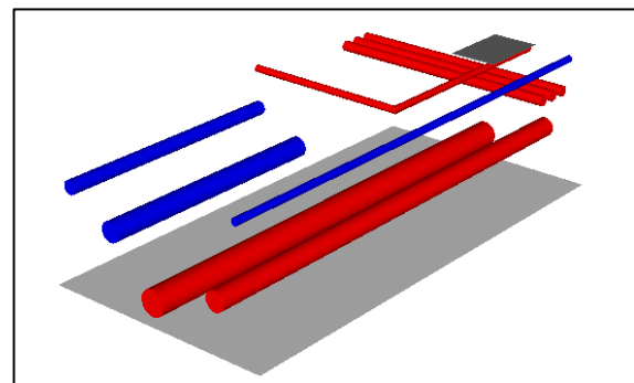
図-2 埋設管配置状況 探査結果3D表示
