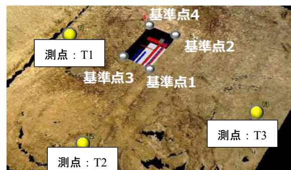
図-4 地上の基準点配置状況
