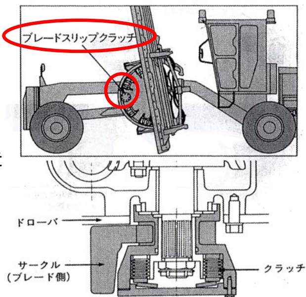
乾式タイプ
