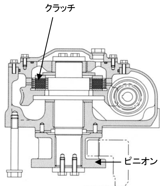
湿式タイプ
