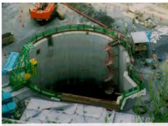
写真-2 奥津第二発電所立坑
