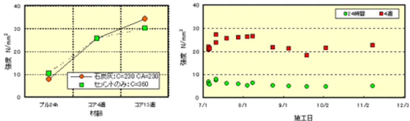
図-1 奥津第二発電所立坑における「EPショット-D工法」の結果
